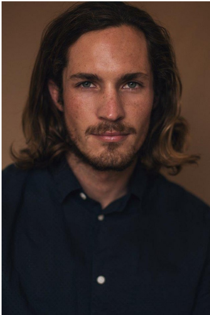
Devin
